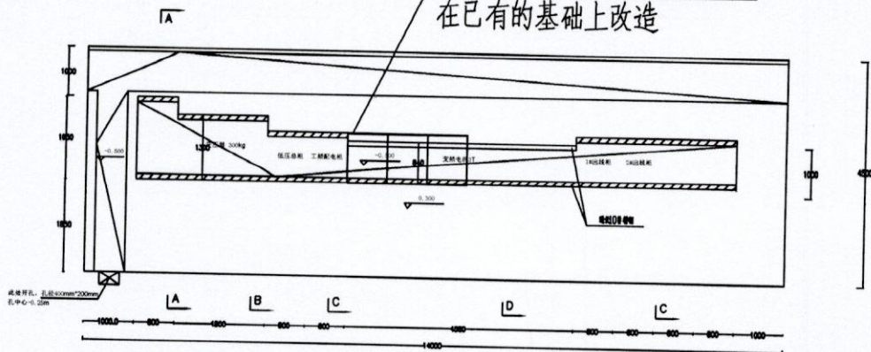
新增三台配电柜基础布置图
