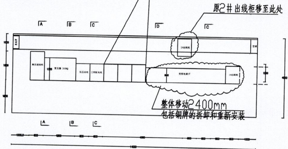
新增三台配电柜基础布置图
