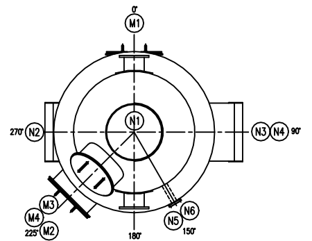
管口方位图 1:20
